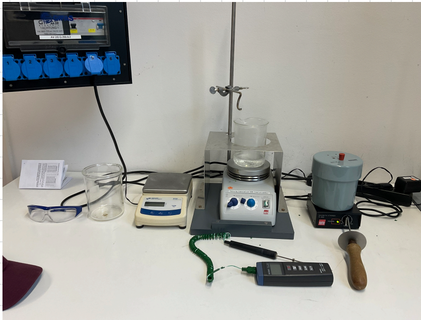
Abb. 3.1: Messaufbau
